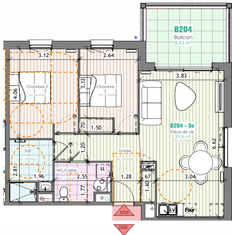
Plan du logement B204 (1 : 100)
