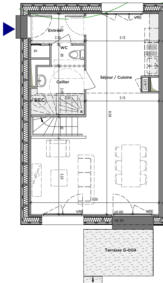
PLAN REZ-DE-CHAUSSEE
