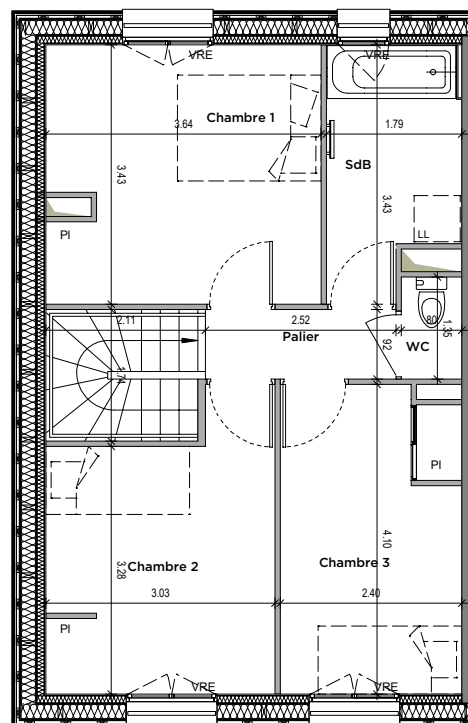
PLAN ETAGE
