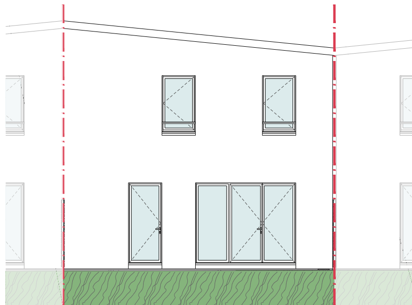
Façade SUD
