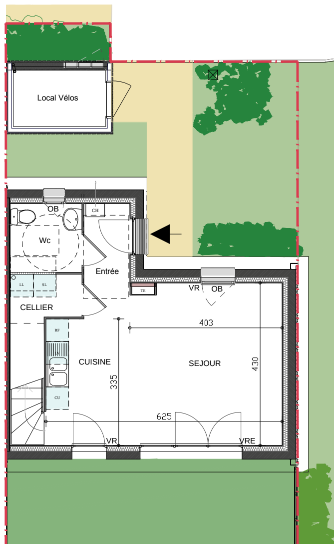
REZ DE CHAUSSEE
