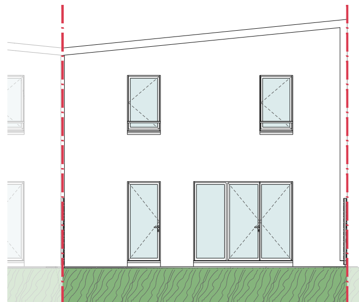
Façade SUD
