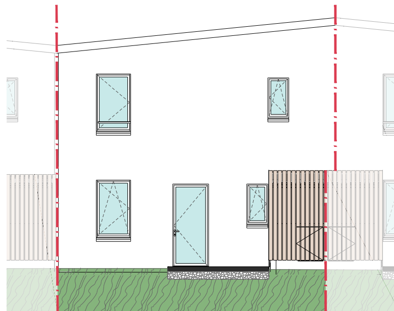
Façade NORD
