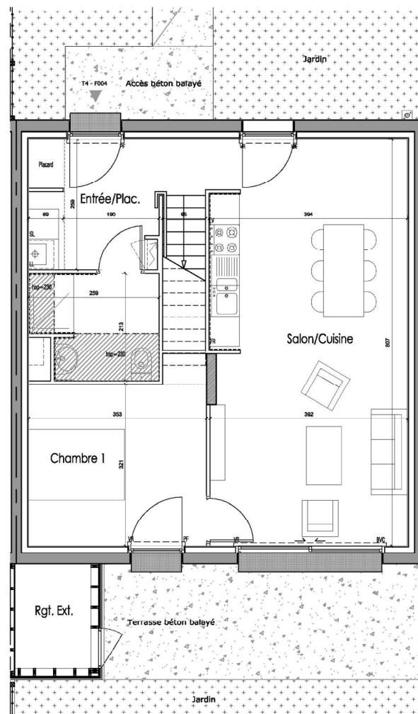
Plan RDC
