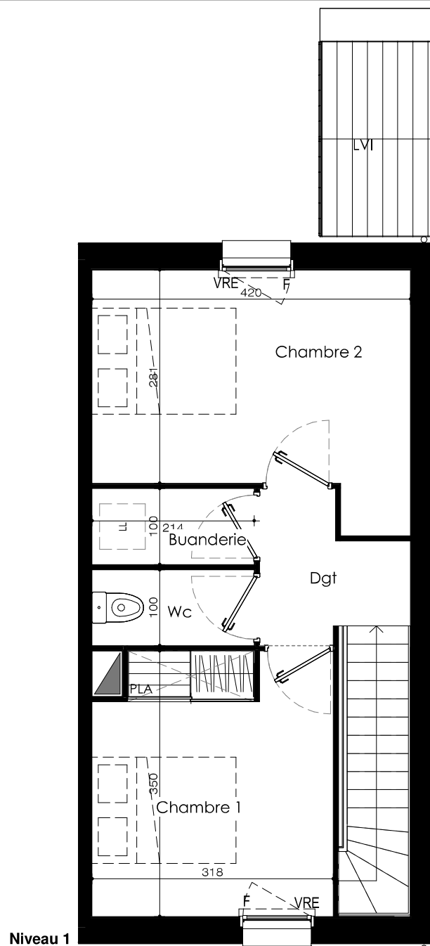
Niveau 1
