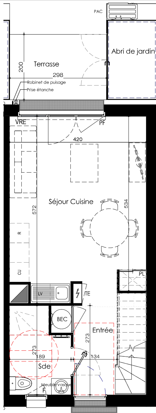
Niveau RDC
