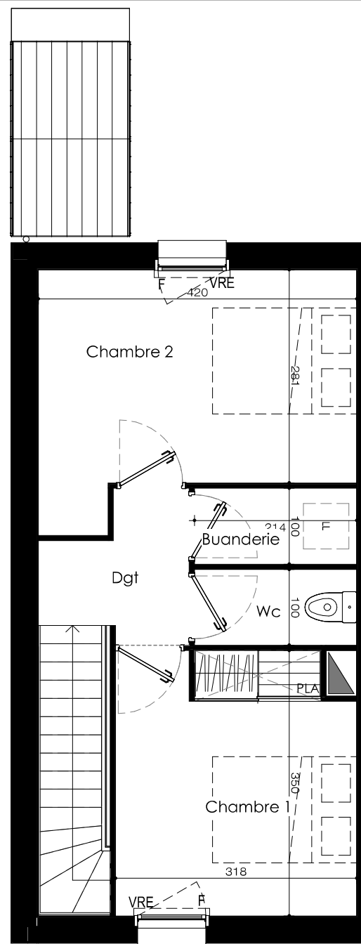
Niveau 1
