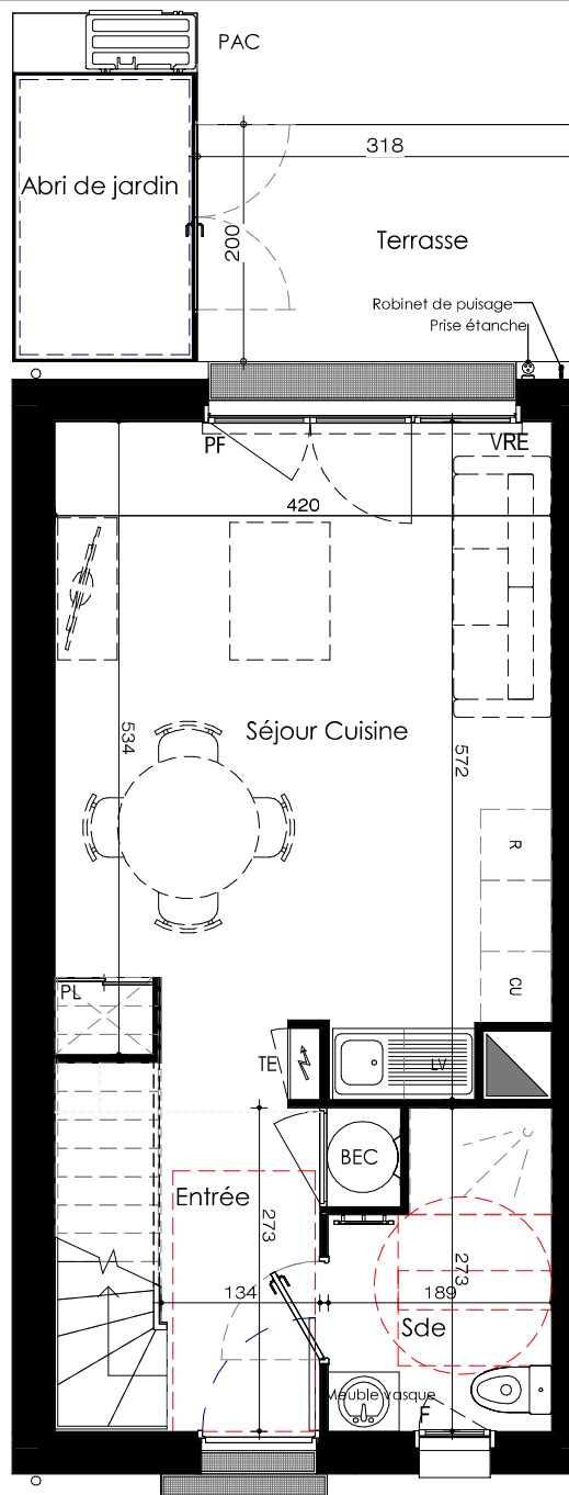
Niveau RDC
