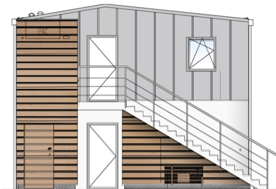
Façade terrasse
