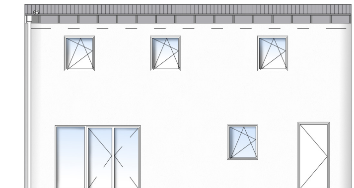
Façade jardin
