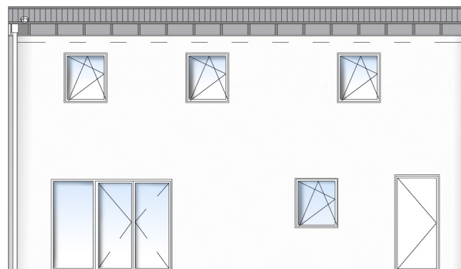
Façade jardin
