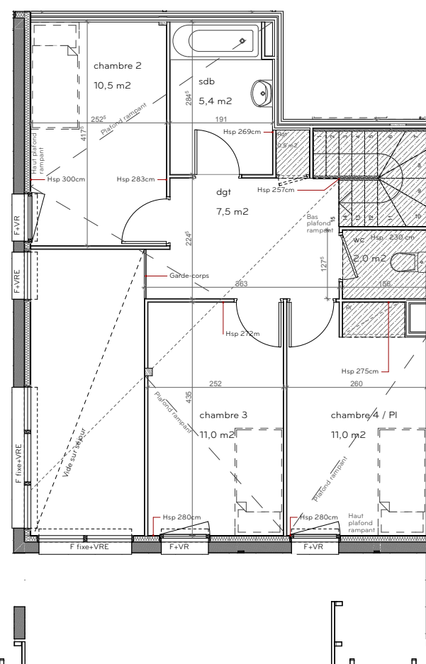
Niveau R+2
