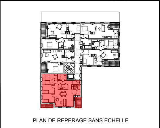
BATIMENT LOGEMENT NIVEAU TYPE 01 205 R+2 T4
