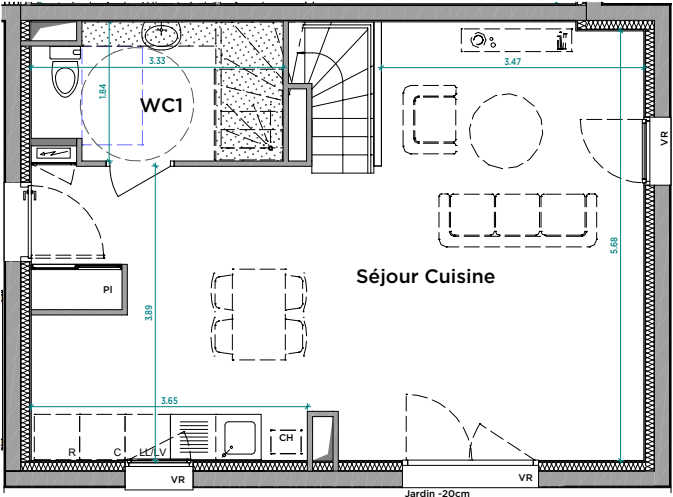
Plan RdC
