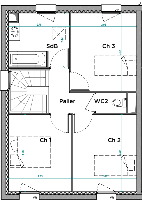
Plan Etage
