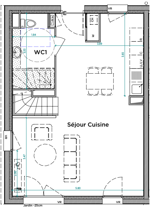
Plan RdC
