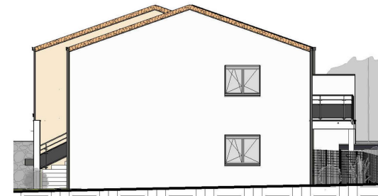
Elévation Ouest Ech : 1 : 150
