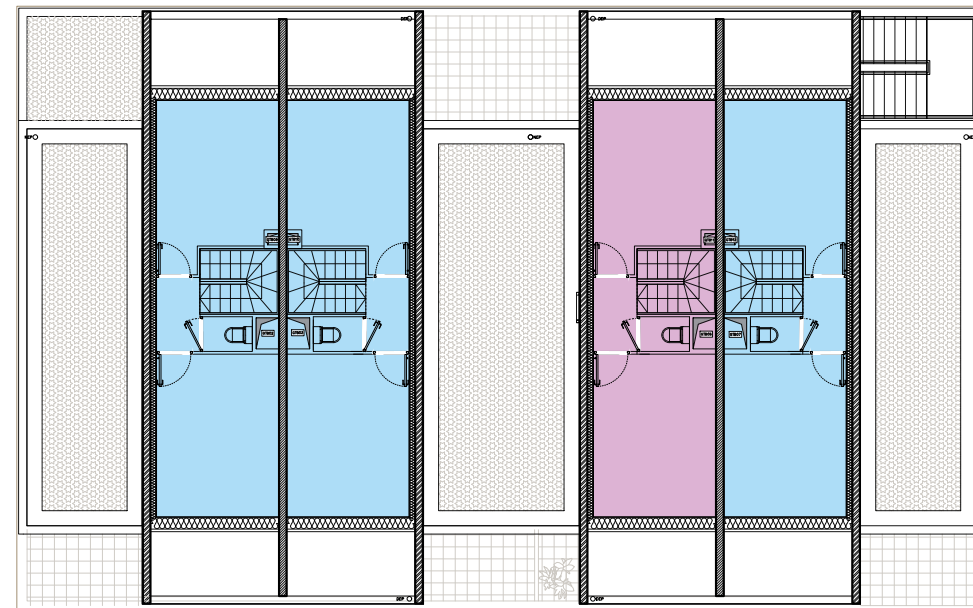
PLAN R+2+C
