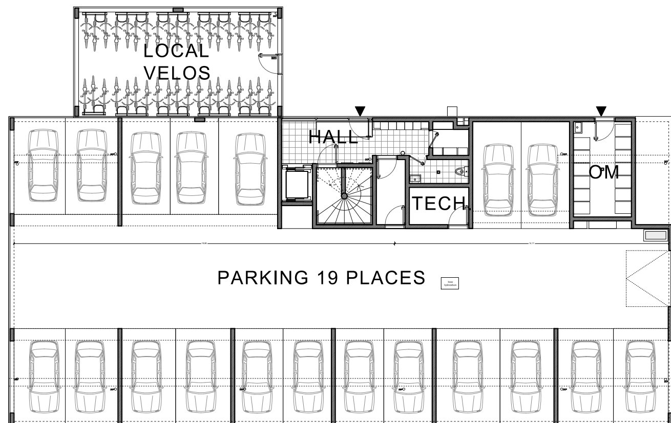
PLAN RDC
