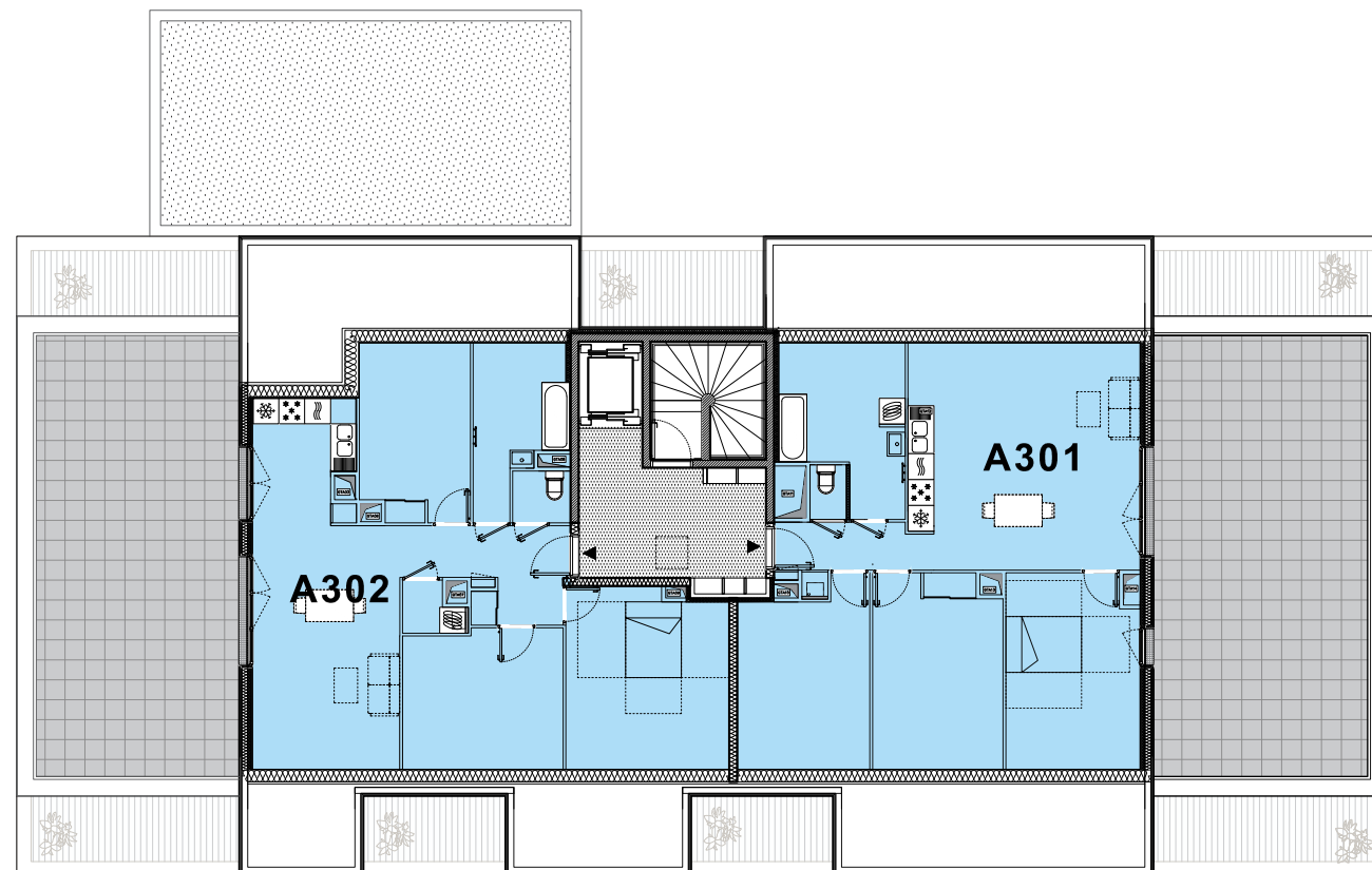
PLAN R+2+C
