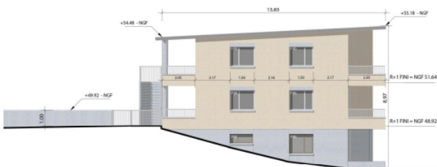
FACADE OUEST
